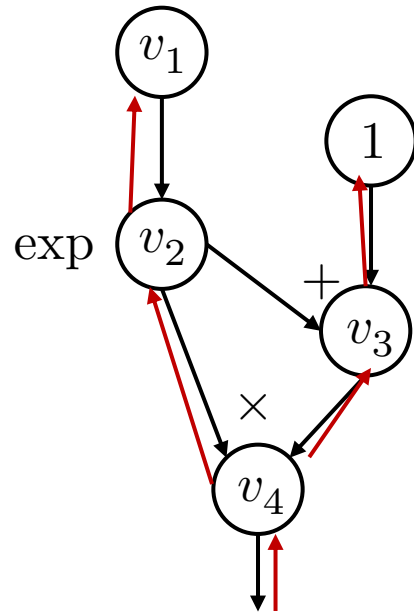
Backprop
